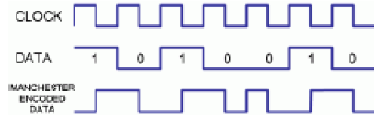
The OOK modulation scheme uses Manchester Coding
